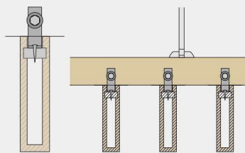
天花板鋼管工法
