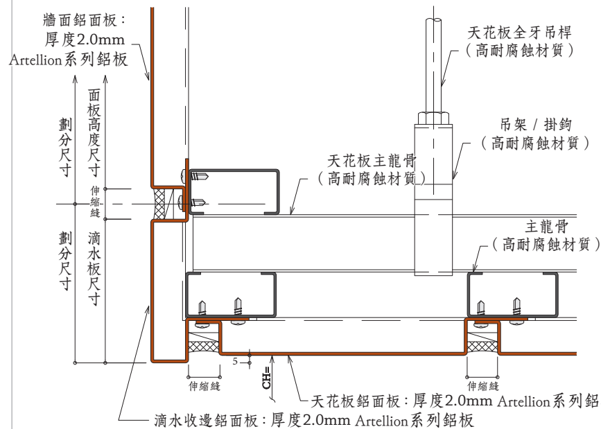
窗台下緣滴水與天花板銜接
