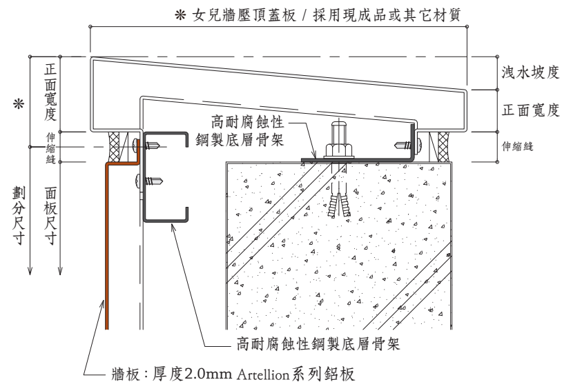
女兒牆壓頂 / 女兒牆蓋板收頭
