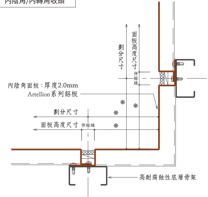
內陰角 / 內轉角收頭
