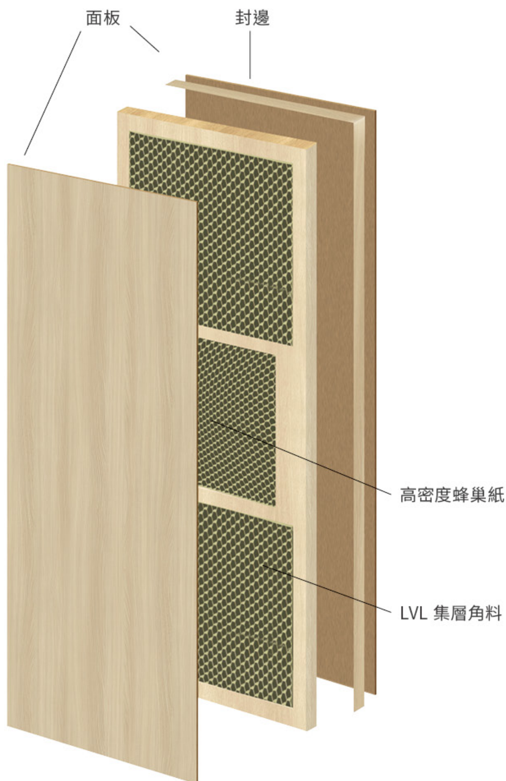
結構示意圖
