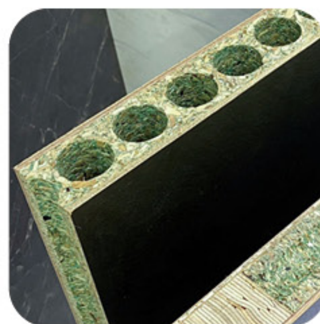
橋洞力學板
