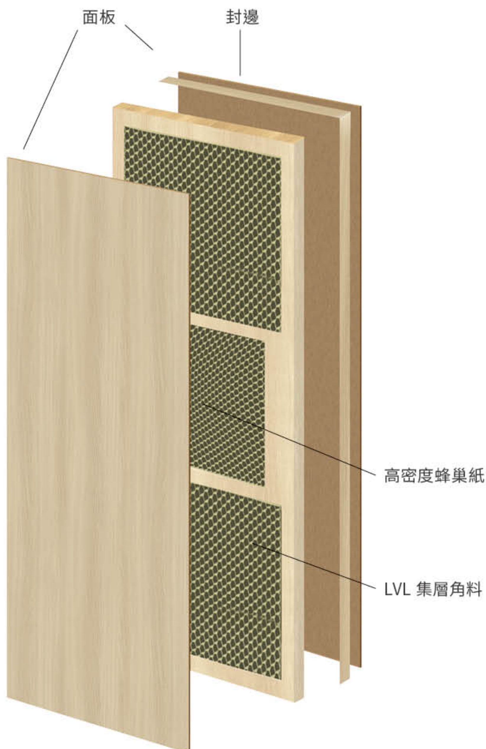
結構示意圖
