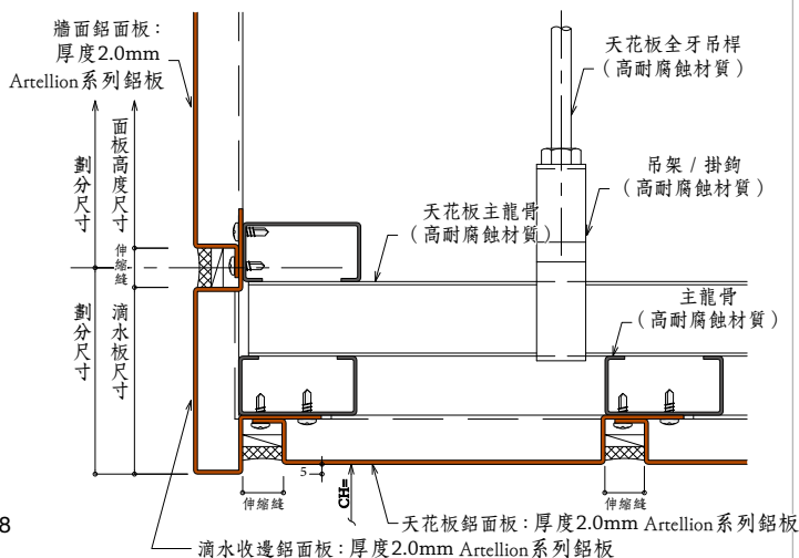
窗台下緣滴水與天花板銜接
