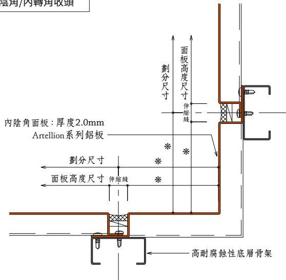
內陰角/內轉角收頭
