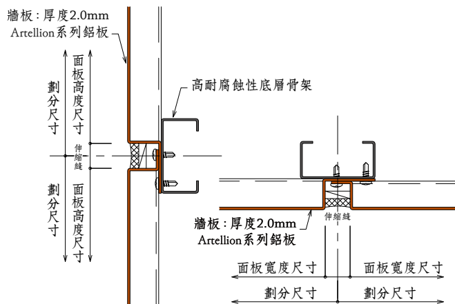
中間伸縮縫收頭
