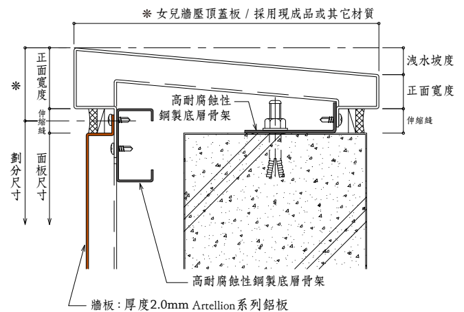
女兒牆壓頂 / 女兒牆蓋板收頭
