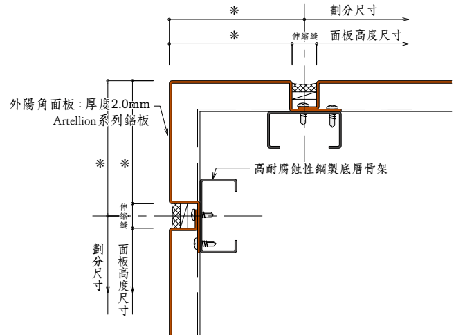
外陽角 / 外轉角收頭
