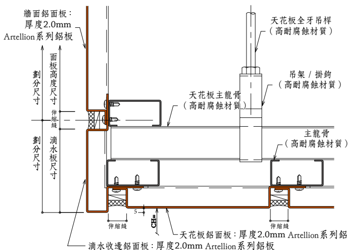
窗台下緣滴水與天花板交接
